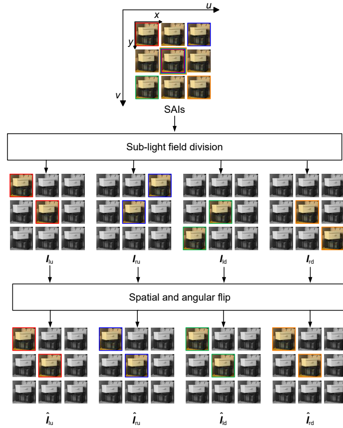
图2 子光场划分和空间角度翻转, 以 3×3 为示例
