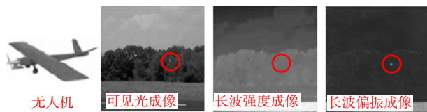
图13 小型遥控无人机长波红外偏振成像与可见光、红外强度成像结果对比 [57]
