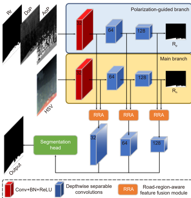
图 18 偏振识别网络示意图。偏振导向分支和主分支与道路区域特征模块感知融合,
