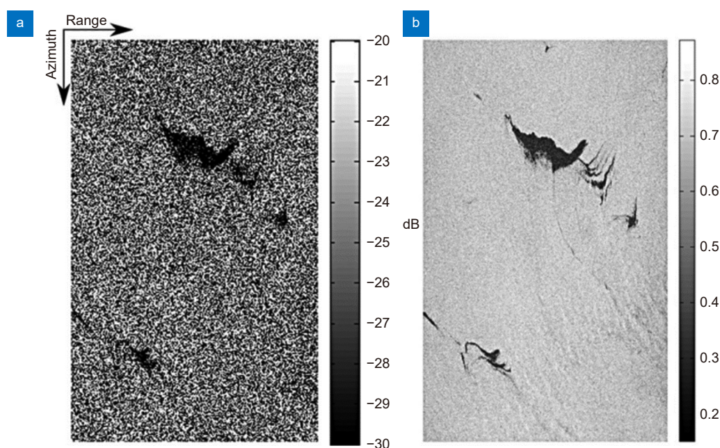
图 19 传统红外热成像和偏振成像海面漏油检测对比 [53]
