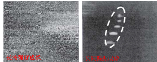
图15 地雷长波红外偏振成像与红外强度成像结果对比 [59]
