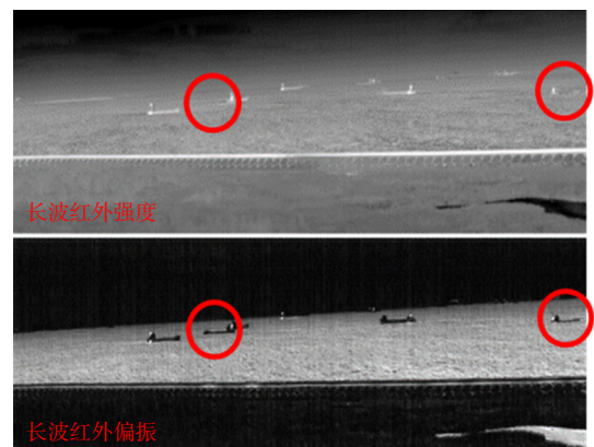
图16 水面舰船目标长波红外偏振成像与红外强度成像结果对比
