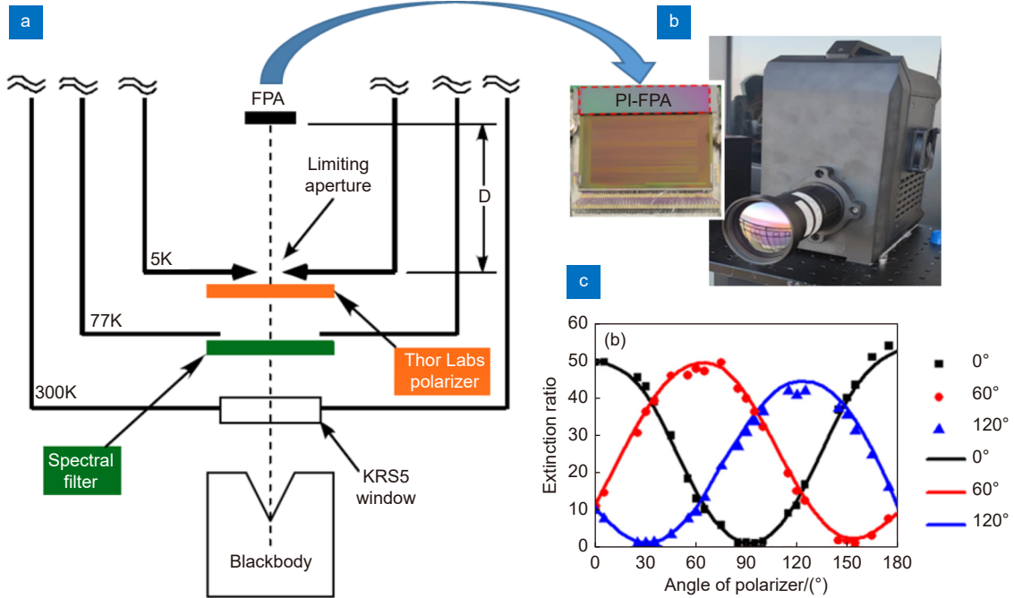
图 11 (a) 偏振集成探测器测试系统示意图 [20] ; (b) 512×4×3 制冷型 InAs/GaSb 超晶格长波红外偏振集成焦平面芯片及组件; (c) 组件消光比测试 [39]
