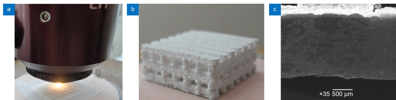
图 7 生物陶瓷支架激光制造 [36] 。(a) 激光沿着预定路径选择性地烧结 \beta -TCP 粉末; (b) 多孔 \beta -TCP 生物陶瓷支架的宏观形态; (c) 单个烧结路径的微观结构
