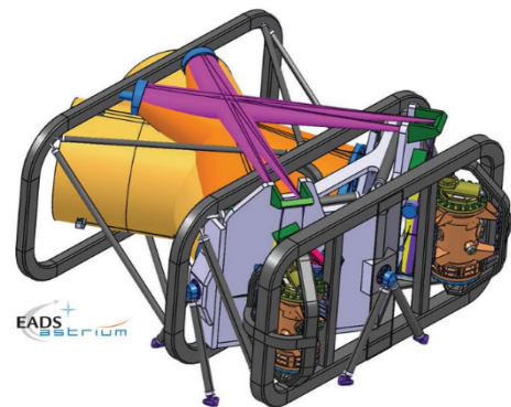
图 15 离轴视场内指向望远镜构型 (望远镜交叉布置) [43]
