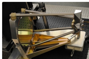
图 3 NASA 与佛罗里达大学联合研制的望远镜原理样机 [24]
