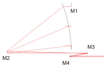
图 2 离轴四反光学系统布局 [11]
