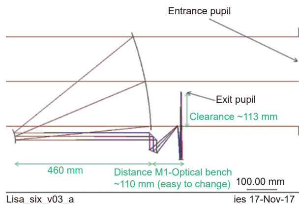
图 5 以柯尔施系统为基础的离轴六反光学系统布局 [25]
