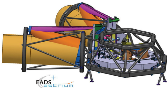
图 14 离轴视场内指向望远镜构型 [43]
