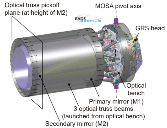
图 13 离轴望远镜构型 [28]
