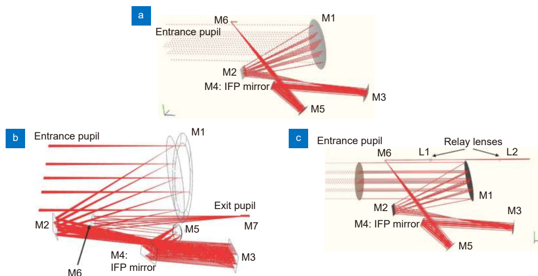
图 7 视场内指向光学系统 [19]
