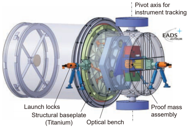
图 12 同轴望远镜构型 [37]
