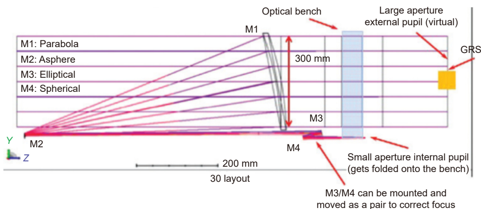
图 4 以卡塞格林系统为基础的离轴四反光学系统布局 [25]
