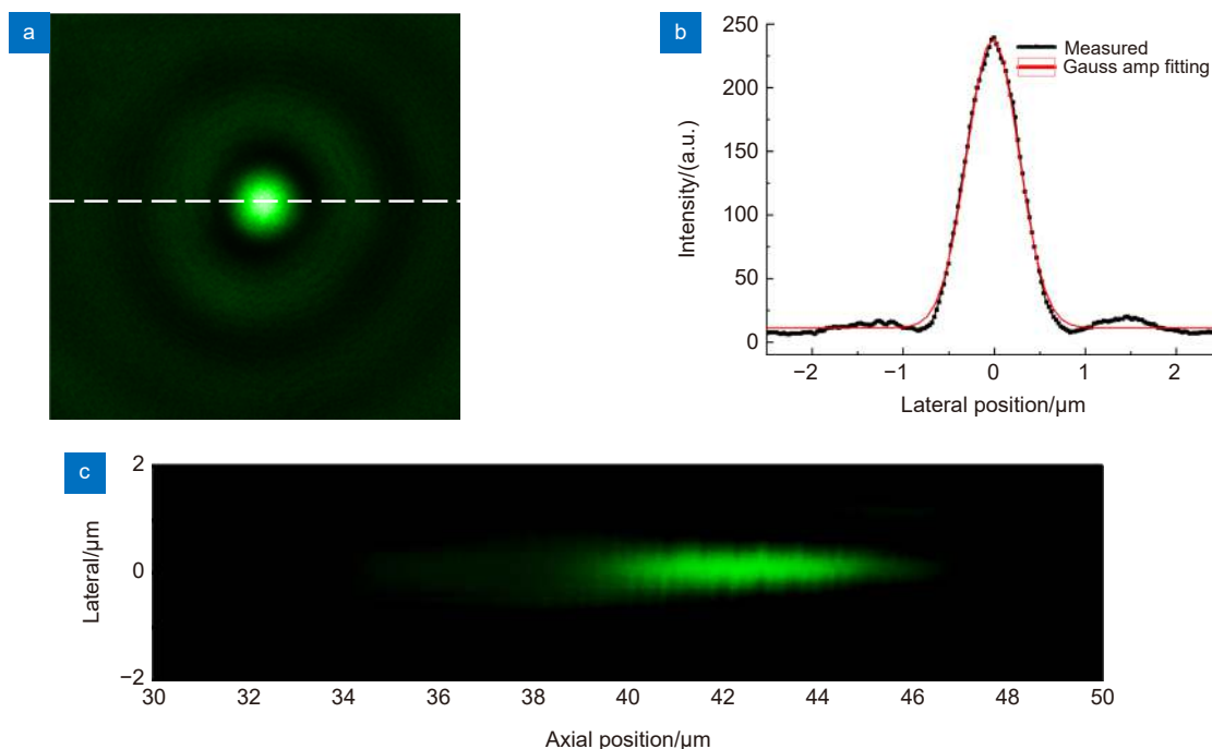
图 4 单层菲涅尔波带片在 535\text{ nm} 波长处的聚焦特性。
