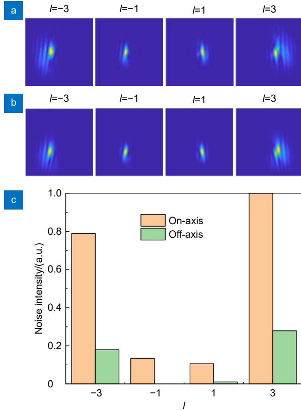
图 5 (a) 同轴与 (b) 离轴系统中不同 OAM 状态 ( l = \pm 1, \pm 3 ) 对应的出射光强分布图; (c) 同轴与离轴系统中不同
