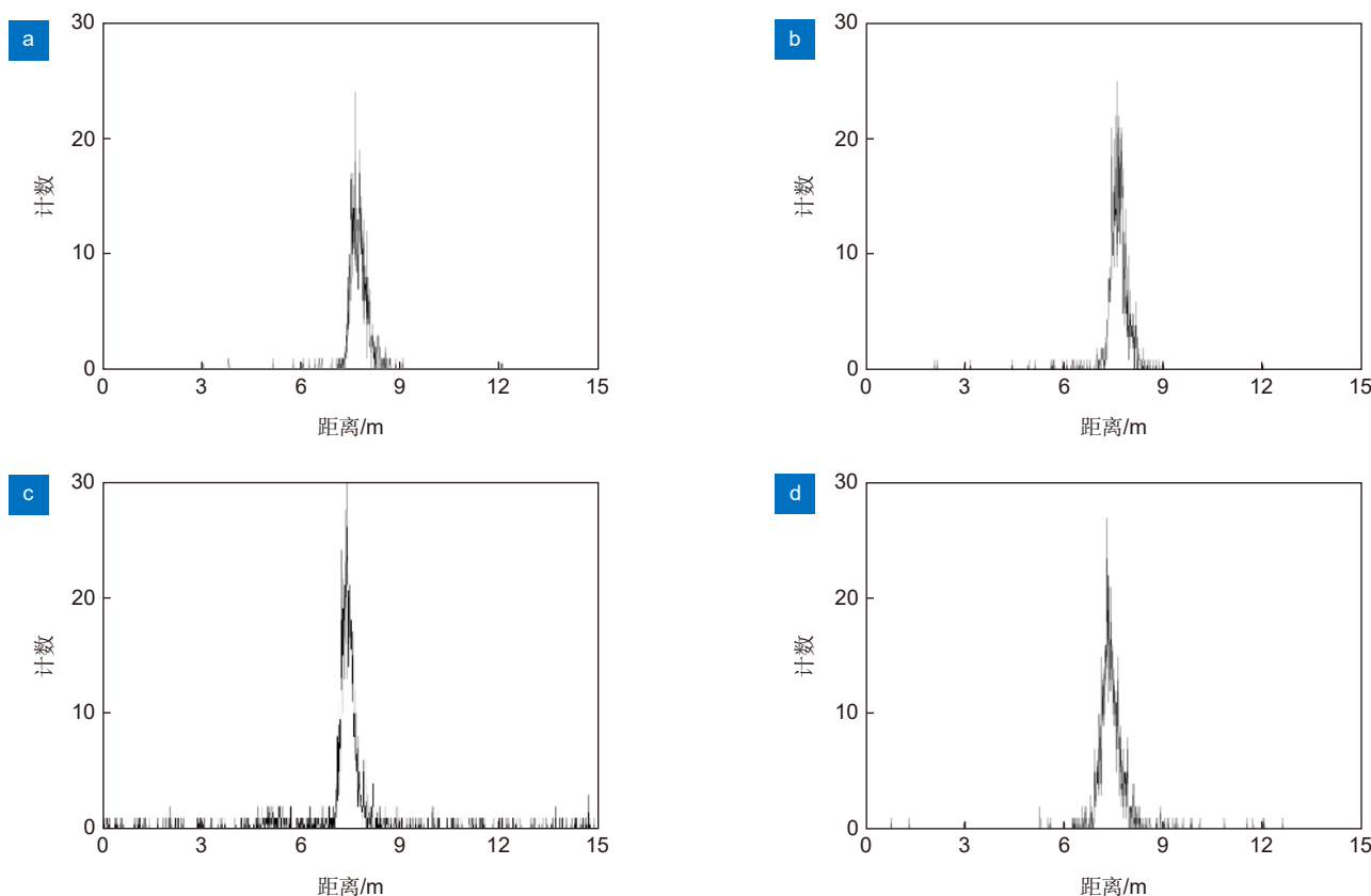
图 10 实验结果。(a) 单模光纤; (b) 单模光纤 (0.5 nm 滤光片); (c) 多模光纤; (d) 多模光纤 (0.5 nm 滤光片)
