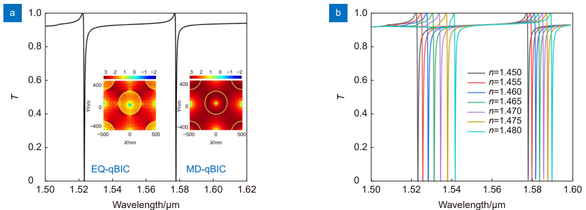
图 2 (a) n=1.450 时超表面的仿真零阶透射谱图 (插图是两个共振模式下的电场分布图); (b) 不同折射率的仿真透射光谱图
