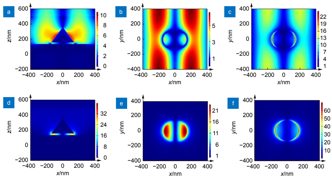
图3 复合结构中两种模式共振波长下的电场分布图。金纳米锥底面半径为 140 nm, 高度为 200 nm, 周期为 800 nm, 背景折射率为 1.30. (a) 和 (d) 为 x - z 平面上的电场分布, (b) 和 (e) 为 \text{SiO}_2 间隔层下表面和 Au 薄膜界面上的电场分布, (c) 和 (f) 为分析物与 \text{SiO}_2 间隔层上表面上的电场分布; (a)、(b)、(c) 为模式 1, (d)、(e)、(f) 为模式 2
