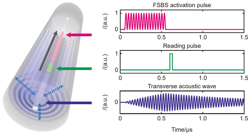
图 11 基于本地光相位追溯技术的分布式 F-SBS 测量。激发光与探测光不仅在波长上不同, 也在时间上区分 [36]
