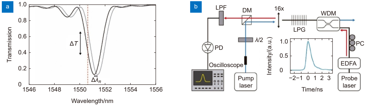
图 10 LPG 用于解调 F-SBS。(a) 原理示意图; (b) 实验装置图 [45]
