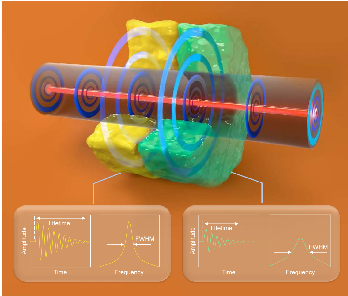
图 5 F-SBS 用于声阻抗传感的原理示意图
