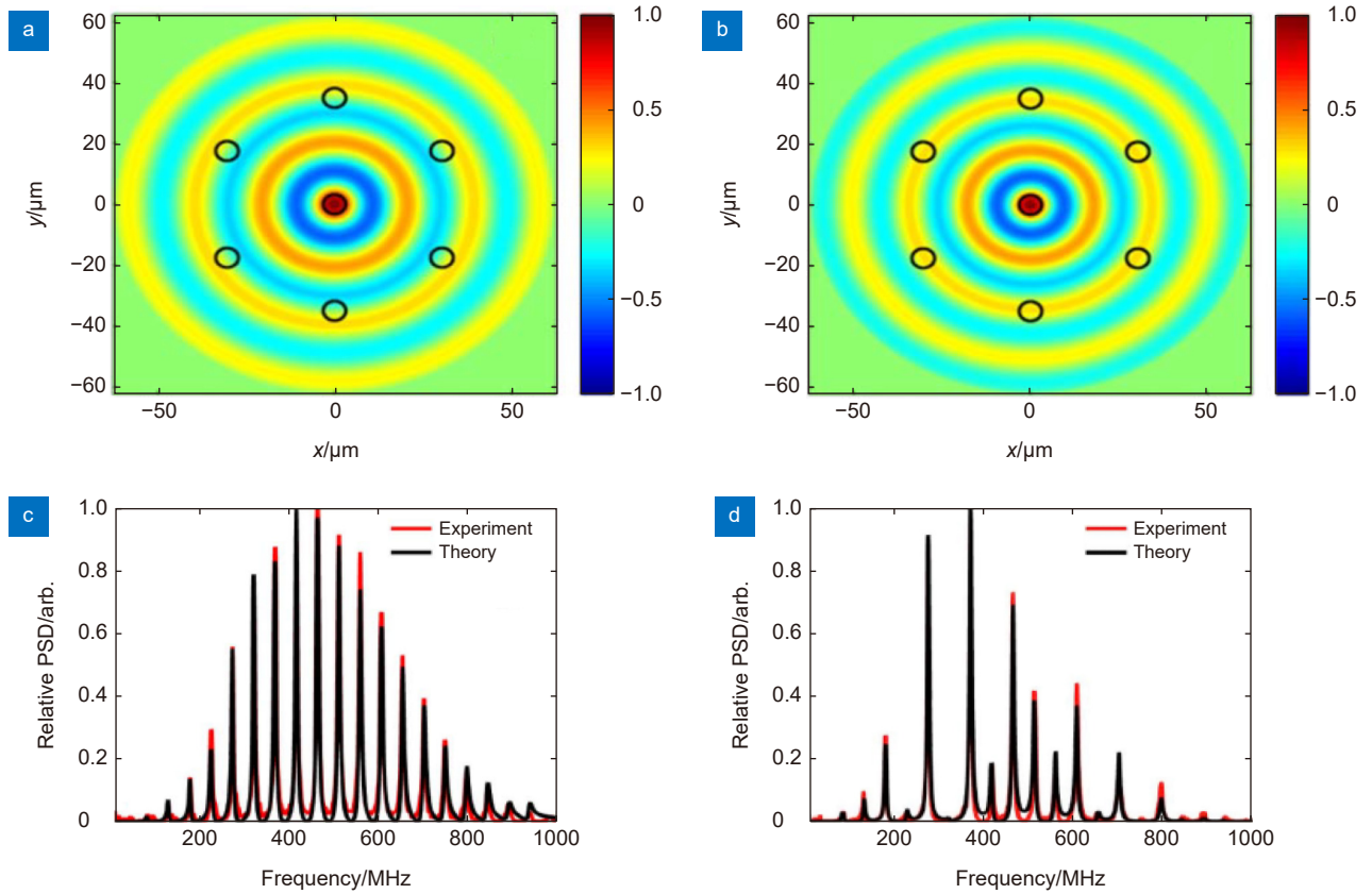
图 8 多芯光纤中的 F-SBS。(a), (b) R_{0,7} 和 R_{0,8} 模的位移场分布;
