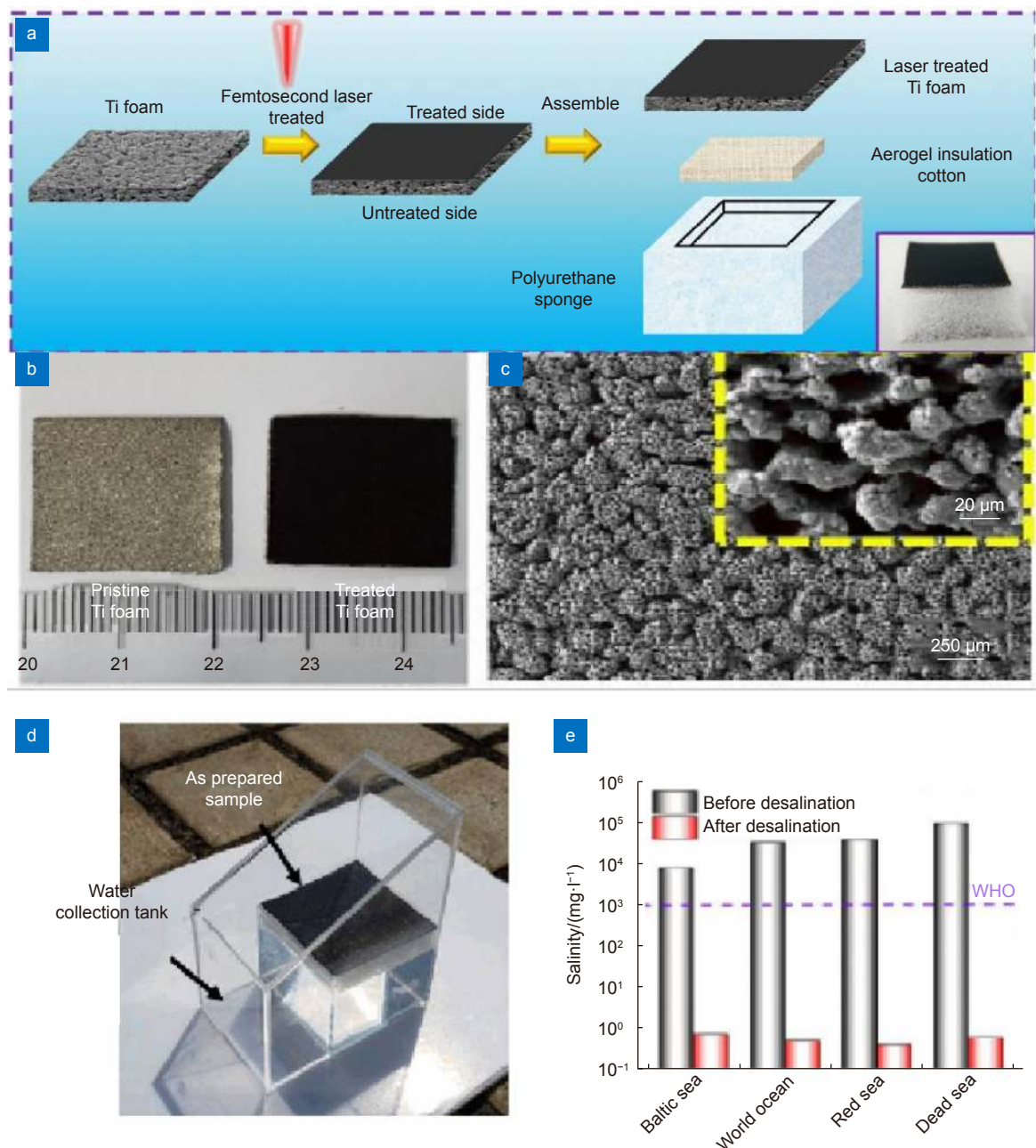
图 7 激光加工的泡沫钛 [94] 。
