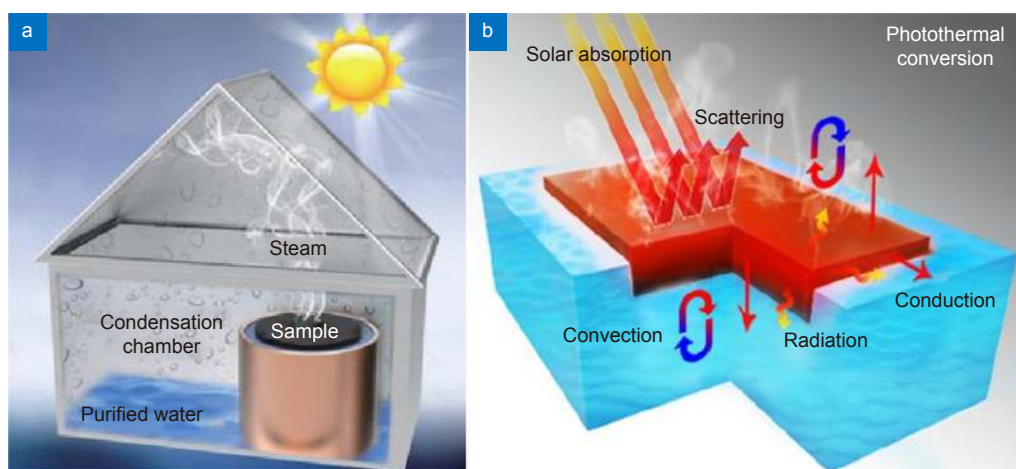
图 2 (a) 太阳能海水淡化实验装置示意图 [65] ; (b) 太阳能海水淡化材料光热转换过程 [66]
