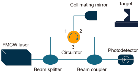
图 1 FMCW 激光测距基本光路图
